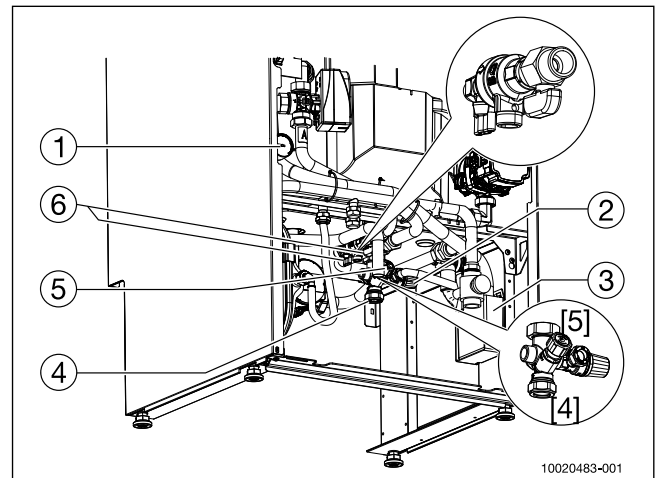
Bild 4 Kopplingsutrymme
