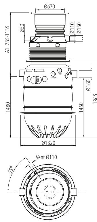
Oleopator P FST 8/800
