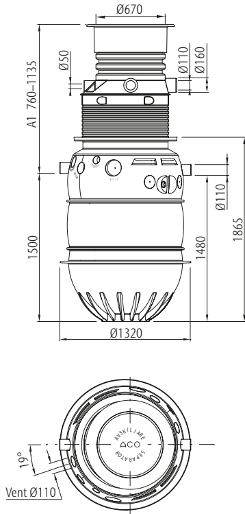
Oleopator P FST 3/900
